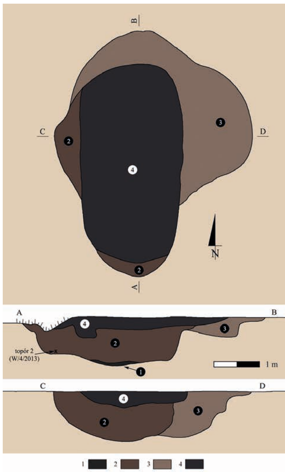
Ryc. 3. Iwiny, gm. Siechnice, stan. 13. Rzut i profil obiektu 295 po doczyszczaniu. Oprac. T. J. Chmielewski na podst. dokumentacji R. Marka i Ł.D. Lisieckiego (2014)
