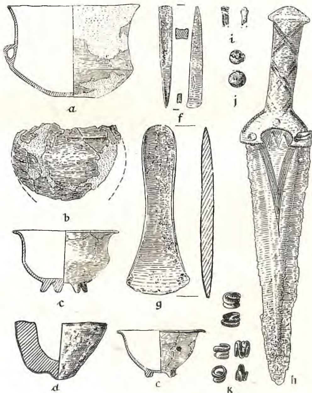
Ryc. 61. Łęki Małe, pow. kościański. Kurhan I. Zawartość grobu D. a.—e. Ceramika, f. Dłuto brązowe, g. Siekierka brązowa, h. Sztylet brązowy, i. Ułamki szpil brązowych, j. Paciorki bursztynowe, k. Złote ozdoby spiralne. a., c., e. w 1/4, b. w 1/2, d., f.—k. w 1/2 w. n. — Fig. 61. Łęki Małe, Tumulus No. I. Contenu de la tombe D. a., c., e. Vases, f. Ciseau en bronze, g. Hache en bronze, h. Poignard en bronze, i. Fragments des épingles en bronze, j. Perles en ambre, k. Pendeloques en or. a., c., e. en 1/4, b. en 1/2, d. f.—k. en 1/2 gr. nat.
