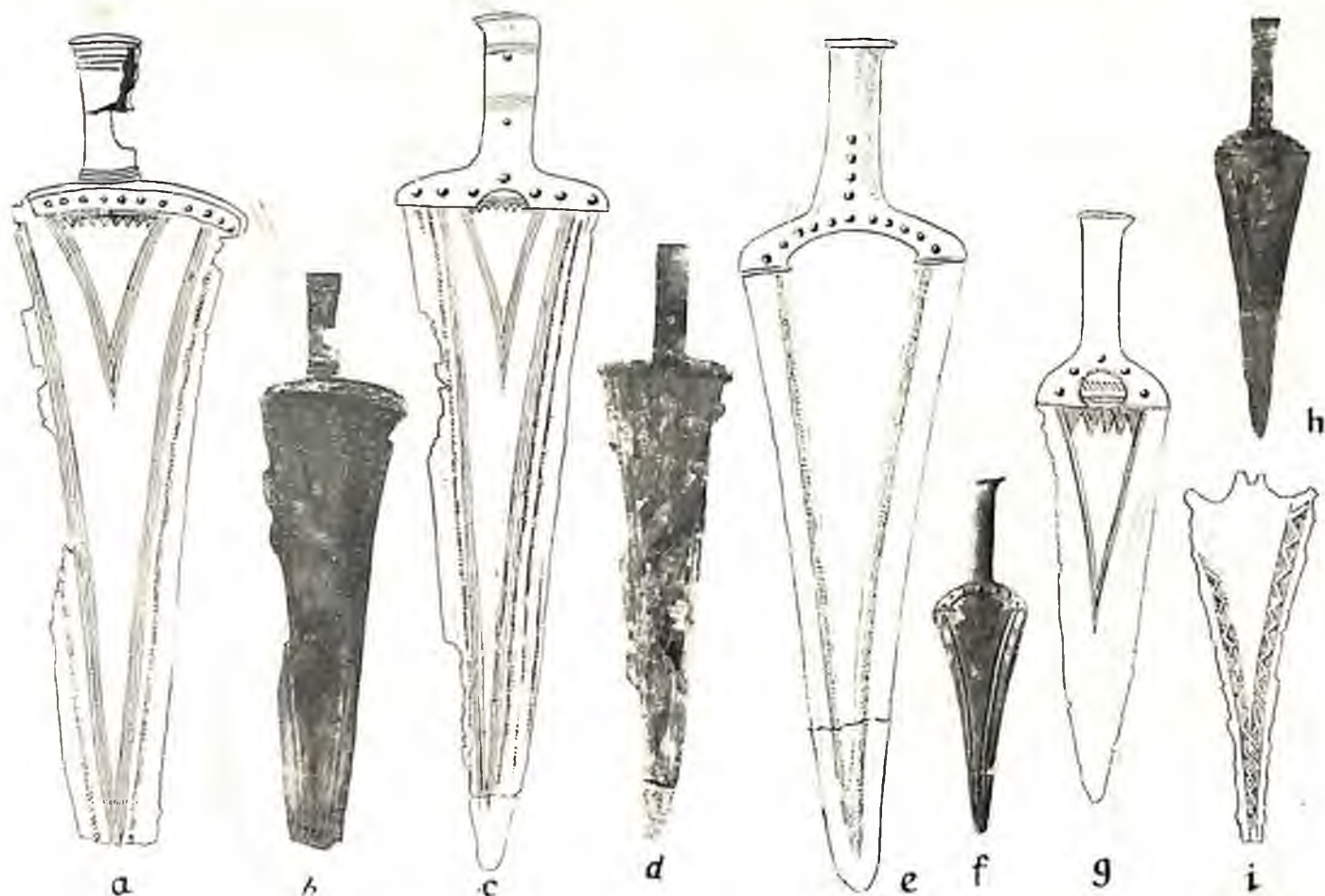
Ryc. 25. Granowo, pow. nowotomyski. Mieczyki i sztylety brązowe ze skarbu. a.—b. Mieczyk, a. w \frac{1}{4} w. n., b. w \frac{1}{6} w. n., c.—d. Mieczyk, c. w \frac{1}{4} , d. w \frac{1}{6} w. n., e. Mieczyk w \frac{1}{4} w. n., f.—i. sztylety, f, h w \frac{1}{6} g, i w \frac{1}{4} w. n. — Fig. 25. Granowo, distr. de Nowy Tomysl, Épées et poignards en bronze d'un dépôt. a.—b. Épée, a. en \frac{1}{4} , b. en \frac{1}{6} gr. nat., c.—d. Épée, c. en \frac{1}{4} , d. en \frac{1}{6} gr. nat., e. Épée \frac{1}{4} gr. nat., f.—i. poignards, f. h. en \frac{1}{6} gr. nat., g. i. en \frac{1}{4} gr. nat.
