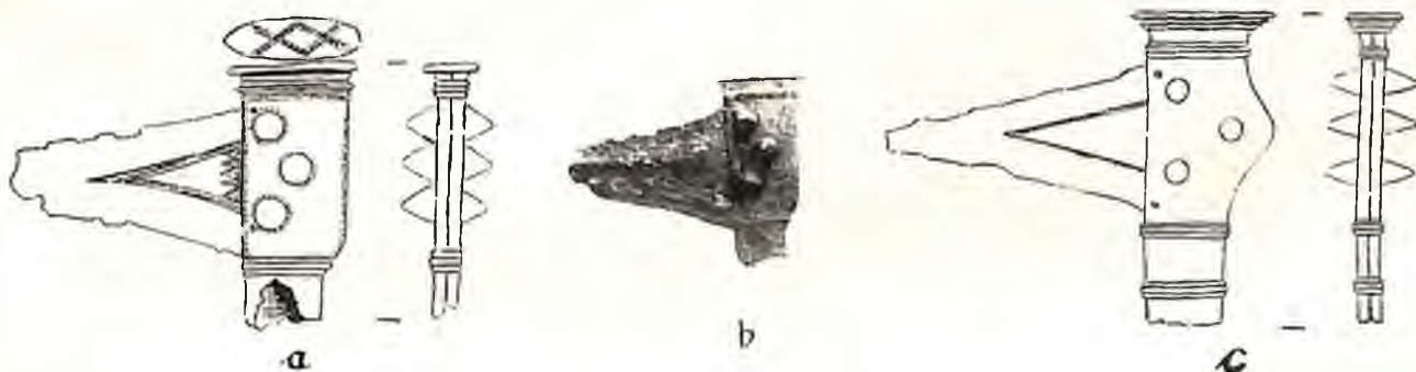
Ryc. 24. Granowo, pow. nowotomyski. Dwa brązowe berła sztyletowe ze skarbu. a—b. Typ wielkopolski, c. Typ brandenbursko-meklemburski. a. i c. w \frac{1}{4} , b. w \frac{1}{6} . — Fig. 24. Granowo, distr. de Nowy Tomyśl. Deux haches-poignards en bronze d'un dépôt. a—b. Type local polonais, c. Type de Brandebourg et Mecklembourg. a. et c. en \frac{1}{4} , b. en \frac{1}{6} gr. nat.
