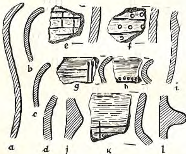
Ryc. 77. Pietrzyków, pow. koniński. Ułamki naczyń 2/3 w. n. — Fig. 77. Pietrzyków, distr. de Konin. Fragments de vases. 2/3 gr. nat.
