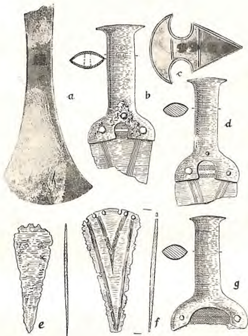
Ryc. 81. Poniec, pow. gostyński. Skarb brązowy. a. Siekierka, b., d.—g. Sztylety, c. Tarczka ozdobna. a., c. w \frac{1}{3} w. n. reszta w \frac{1}{2} w. n. — Fig. 81. Poniec, distr. de Gostyń. Dépôt en bronze. a. Hache, b., d.—g. Poignards, c. Plaque ornemental. a., c. en \frac{1}{3} , le reste en \frac{1}{2} gr. nat.
