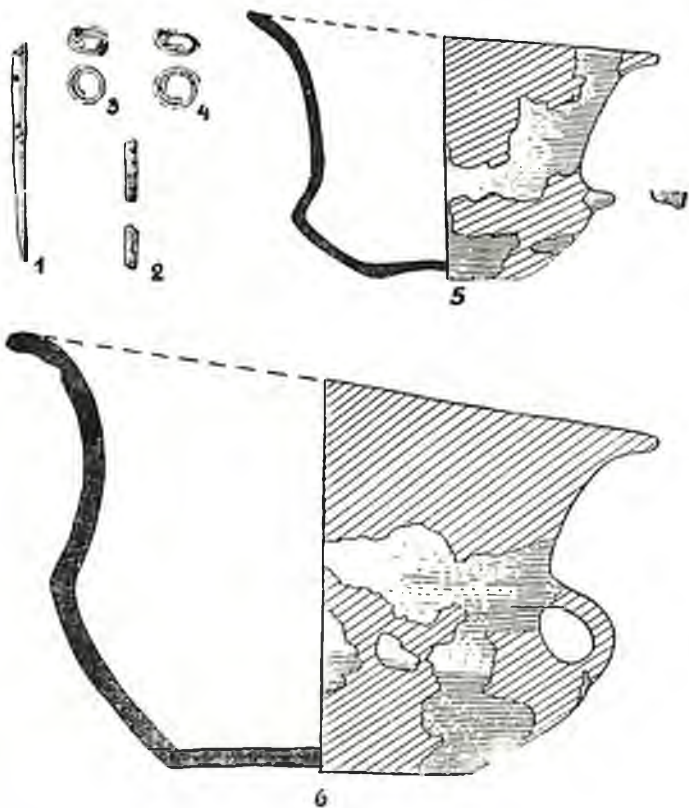
Ryc. 25. Łęki Małe, pow. kościański. Kurhan III. Zespół zabytków z grobu „B.” 1—2. Szpile brązowe, 3—4. Spiralki złote, 5—6. ceramika 1/2 w. n. — Fig. 25. Łęki Małe, distr. de Kościan. Tumulus No III. Mobilier de la tombe „B.” 1—2. Épingles en bronze, 3—4. Anneaux spirals en or, 5—6. Vases en argile. 1/2 gr. nat.
