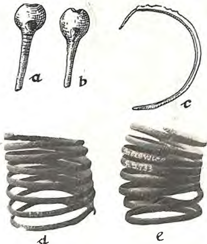
Ryc. 22. Gorszewice, pow. szamotulski. Grób 4 (ogn. nr 50). a—b. Szpile brązowe. W. n. c. Ułamek spiralnej bransolety brązowej. W. n. d—e. Brązowe bransolety spiralne. Ok. 4/5 w. n. — Fig. 22. Gorszewice, distr. de Szamotuły. Tombe No 4. a—b. Épingles en bronze. Gr. nat., c. Fragment d'un bracelet spiral. Gr. nat., d—e. Bracelets spirales. Env. 4/5 gr. nat.
