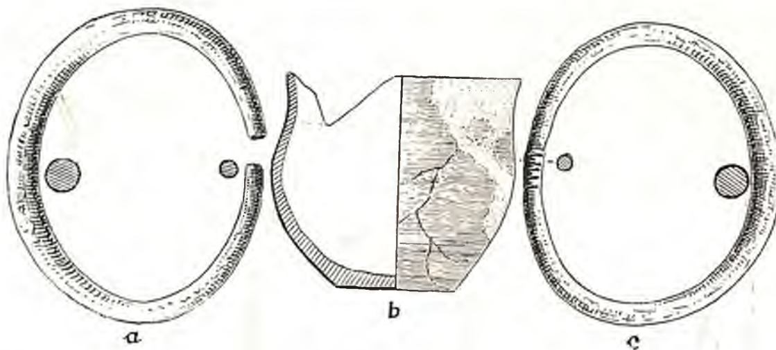
Ryc. 37. Grobia, pow. międzychodzki. Cmentarzysko II, grób 5. a. i c. Naramienniki, b. Naczynie \frac{1}{2} w. n. Fig. 37. Grobia, distr. de Międzychód. II nd cimetière. Tombe No 5. a et c. Brassards, b. Vase \frac{1}{2} gr. nat.
