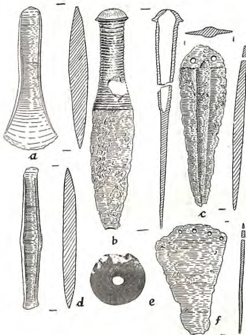
Ryc. 83. Przysieka Polska, pow. kościański. Skarb brązowy. a. Siekierka, b.—c. i f. Sztylety, d. Dłuto, e. Pociorek bursztynowy. a.—d. i f. w \frac{1}{2} w. n., e. w \frac{2}{3} w. n. — Fig. 83. Przysieka Polska, distr. de Kościan. Dépôt. a. Hache en bronze, b.—c. et f. Poignards, d. Ciseau, e. Perle d'ambre. a.—d. et f. en \frac{1}{2} , e. en \frac{2}{3} gr. nat.
