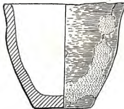
Ryc. 39. Grobia, pow. międzychodzki. Cmentarzysko II, grób 8. Naczynie. \frac{2}{3} w. n. — Fig. 39. Grobia, distr. de Międzychód. II nd cimetière. Tombe No 8. Vase. \frac{2}{3} gr. nat.
