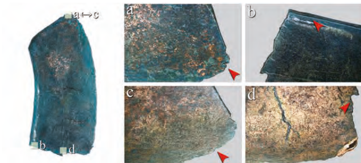
Ryc. 52. Makrostruktury brzytwy typu Biernatki War_6 z Wartosławia, gm. Wronki. Na zdjęciach widoczne są (d) uszkodzenia mechaniczne w postaci pęknięć prawdopodobnie wzdłuż granic ziaren oraz (a, c) wyszczerbienia krawędzi (pow. \times 3,5 ). Oprac. Łukasz Kowalski, Aldona Garbacz-Klempka, fot. Łukasz Kowalski
