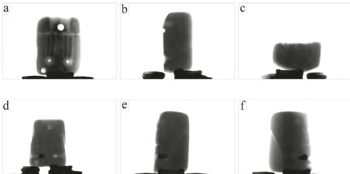
Ryc. 58. Obrazy rentgenowskie kamiennej formy odlewniczej z Wartosławia gm. Wronki. Widoczne są (a) wnęka formy wraz z układem wlewowym dwukanałowym, (d) gniazdo rdzennika, (d) kanały odpowietrzające oraz (a, d) otwory na kołki centrujące. Czytelny jest (d-f) metaliczny czop blokujący kanał formy. Oprac. Łukasz Kowalski, Aldona Garbacz-Klempka, fot. Łukasz Kowalski
