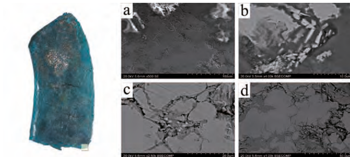
Ryc. 47. Obrazy BSE mikrostruktur brzytwy War_6 z Wartosławia, gm. Wronki. Widoczne są (b, c, d) produkty korozji międzykrystalicznej zachodzącej na granicy ziaren. Skład chemiczny i mikrostruktura wskazują na brąz cynowo - ołowiowy. Obecność ołowiu widoczna w postaci drobnych białych wydzieleń; (a) pow. \times 500 , (d) pow. \times 1000 , (c) pow. \times 2500 , (b) pow. \times 4000 . Oprac. Łukasz Kowalski, Aldona Garbacz-Klempka, fot. Łukasz Kowalski
