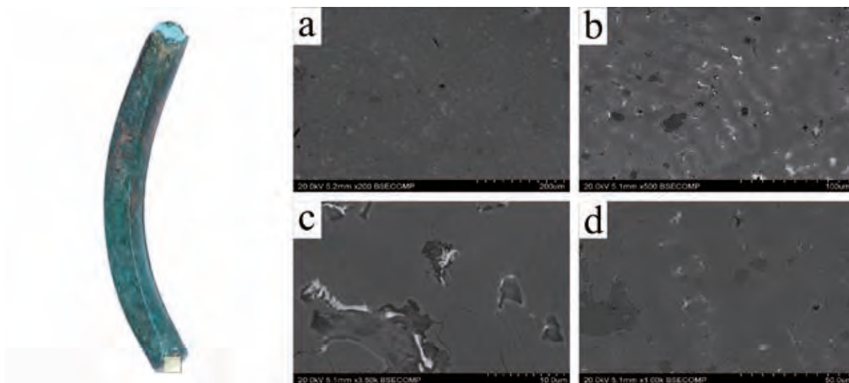
Ryc. 49. Obrazy BSE mikrostruktur pręcika War_8 z Wartosławia, gm. Wronki. Widoczna jest struktura dendrytyczna roztworu stałego niklu i arsenu w miedzi. W przestrzeniach pomiędzy dendrytami widoczne są fazy międzymetaliczne zawierające miedź, arsen i antymon oraz małe białe wydzielania ołowiu. Struktura dendrytyczna dowodzi, że pręcik był odlewany, a zniekształcenie faz międzymetalicznych, dowodzi dodatkowo że przedmiot był przerabiany plastycznie; (a) pow. \times 200 , (b) pow. \times 500 , (d) pow. \times 1000 , (c) pow. \times 3500 . Oprac. Łukasz Kowalski, Aldona Garbacz-Klempka, fot. Łukasz Kowalski
