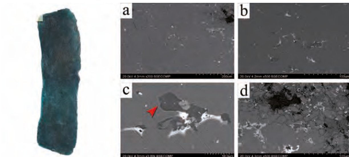
Ryc. 50. Obrazy BSE mikrostruktur brzytwy War_9 z Wartosławia, gm. Wronki. Ośnowę stopu tworzy miedź z cyną i arsenem, a w niej dość liczne i rozległe (a) białe skupiska ołowiu, który wykazuje z miedzią brak rozpuszczalności. Widoczne są (d) granice ziaren, a na granicach produkty korozji o charakterze tlenkowym. Lokalnie występują (c) wydzielania siarczków; (a) pow. \times 200 , (b, d) pow. \times 500 , (c) pow. \times 3000 . Oprac. Łukasz Kowalski, Aldona Garbacz-Klempka, fot. Łukasz Kowalski
