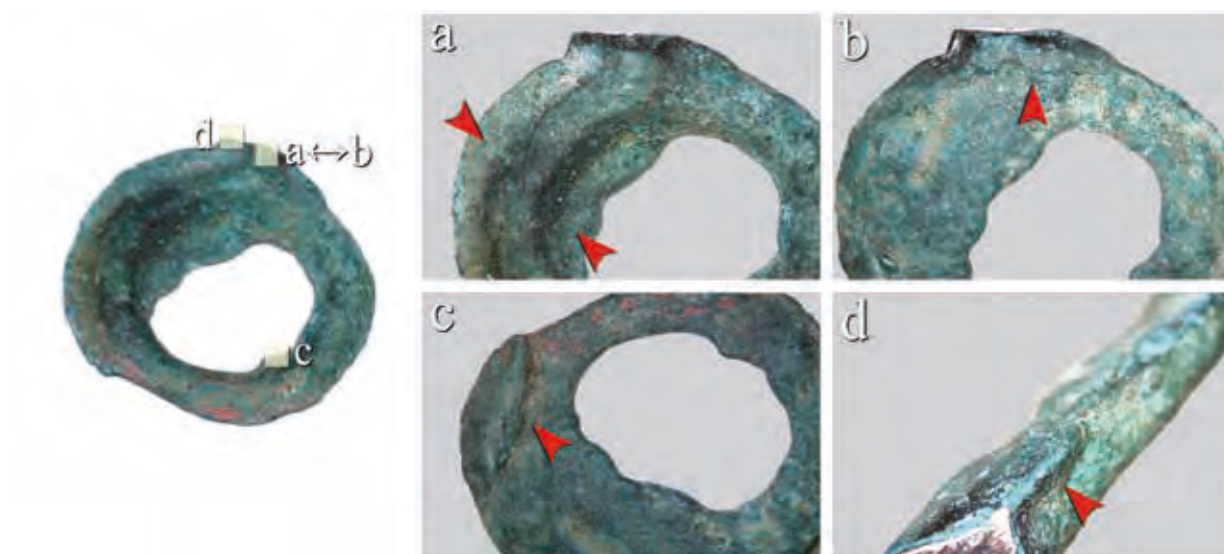
Ryc. 53. Makrostruktury kółka War_7 z Wartosławia, gm. Wronki. Na zdjęciach widoczne są (a) zalewki na płaszczyźnie podziału formy od strony wewnętrznej i zewnętrznej kółka oraz (c) ślady po układzie wlewowym (pow. \times 3,5 ). Oprac. Łukasz Kowalski, Aldona Garbacz-Klempka, fot. Łukasz Kowalski
