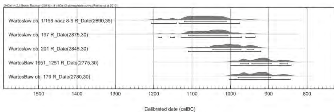
Ryc. 60. Wyniki kalibracji wieków ^{14}\text{C} próbek z Wartosławia. Oprac. Tomasz Goslar
