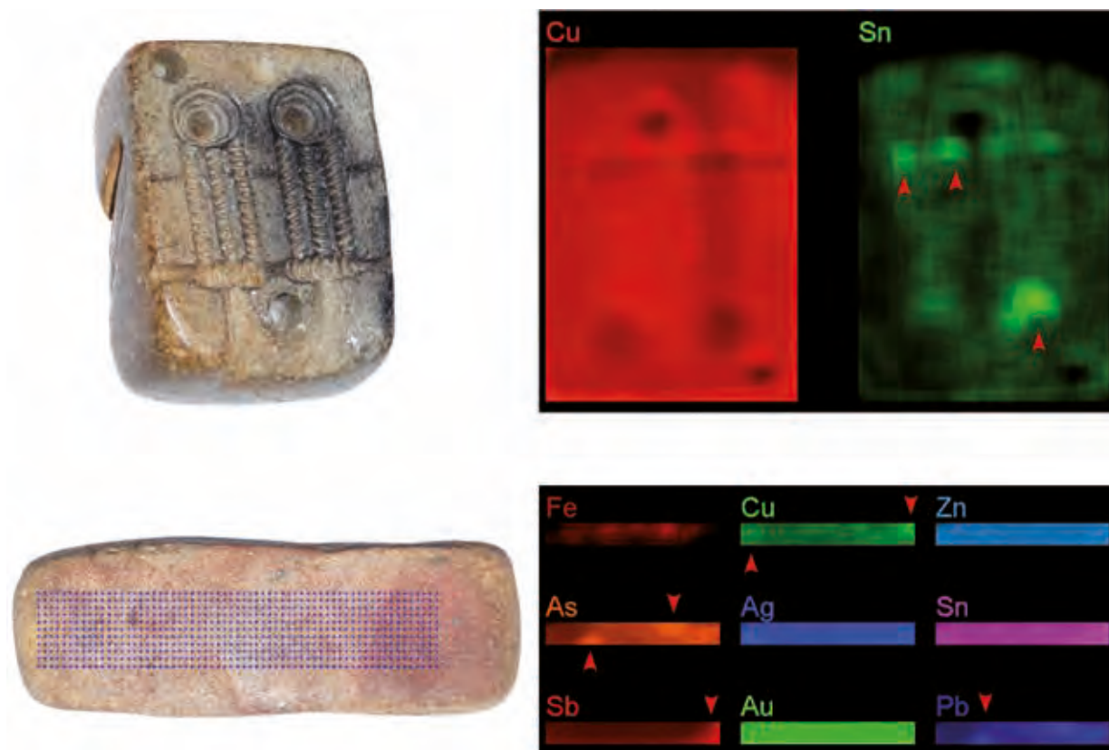
Ryc. 45. Rozkład pierwiastków metalicznych na powierzchniach połówki formy odlawniczej War_13 i gładzika War_16 z Wartosławia, gm. Wronki. Oprac. Łukasz Kowalski, Aldona Garbacz-Klempka, fot. Łukasz Kowalski
