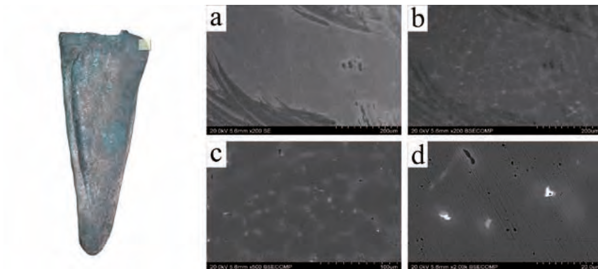
Ryc. 46. Obrazy BSE mikrostruktur fragmentu sierpa War_1 z Wartosławia, gm. Wronki. Na tle ciemnych dendrytów roztworu stałego cyny i niklu w miedzi widoczne są w przestrzeniach międzydendrytycznych jaśniejsze wydzielania eutektoidu zawierającego miedź i cynę (b i c) oraz białe wydzielania ołowiu (d); (a, b) pow. \times 200 , (c) pow. \times 500 , (d) pow. \times 2000 . Oprac. Łukasz Kowalski, Aldona Garbacz-Klempka, fot. Łukasz Kowalski
