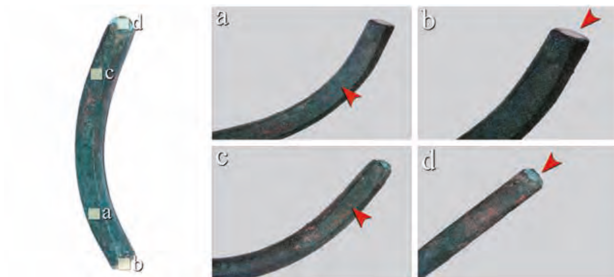
Ryc. 54. Makrostruktury pręcika War_8 z Wartosławia, gm. Wronki. Na zdjęciach widoczny jest pręt po odlaniu i po przeróbce plastycznej (pow. \times 3,5 ). Oprac. Łukasz Kowalski, Aldona Garbacz-Klempka, fot. Łukasz Kowalski
