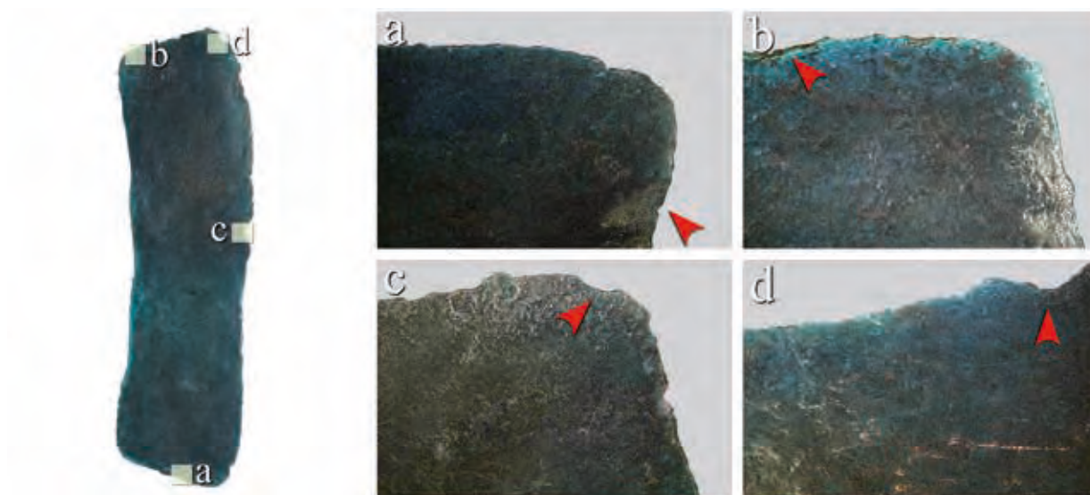
Ryc. 55. Makrostruktury brzytwy typu Biernatki War_9 z Wartosławia, gm. Wronki. Na zdjęciach widoczne są uszkodzenia mechaniczne i wynikające z procesów korozyjnych (pow. \times 3,5 ). Oprac. Łukasz Kowalski, Aldona Garbacz-Klempka, fot. Łukasz Kowalski
