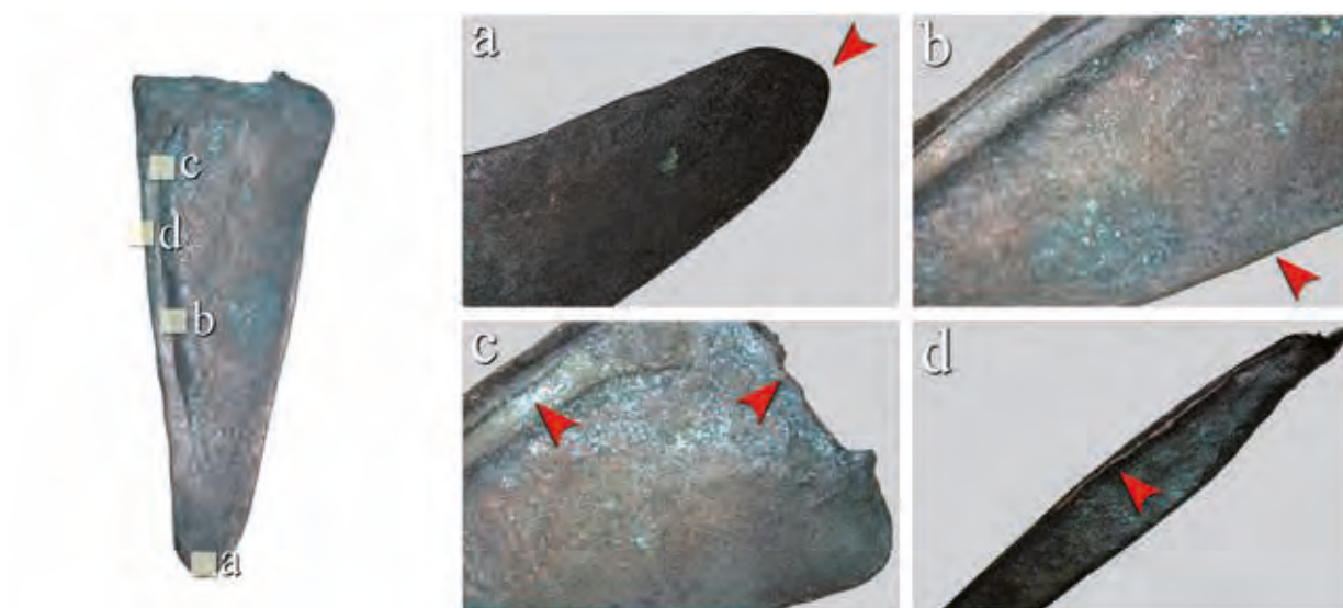
Ryc. 51. Makrostruktury fragmentu sierpa War_1 z Wartosławia, gm. Wronki. Na zdjęciach widoczne są powierzchnie pozbawione wad odlewniczych, które nie były poddawane przeróbce plastycznej (pow. \times 3,5 ). Oprac. Łukasz Kowalski, Aldona Garbacz-Klempka, fot. Łukasz Kowalski
