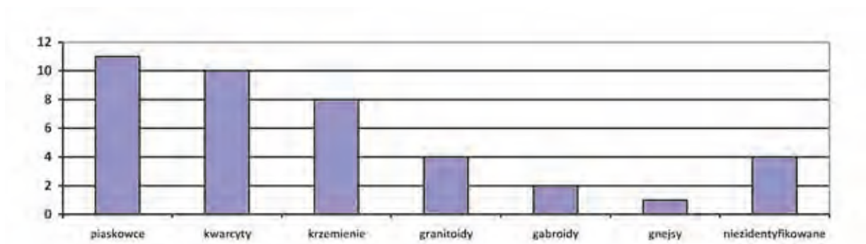
Ryc. 43. Rozkład ilościowy surowców skalnych zastosowanych do wykonania przedmiotów kamiennych w Wartosławiu ze zbioru z badań w 2009 roku. Oprac. Małgorzata Szczepaniak
